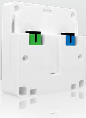
84179716 FTTH-0F-BASE-PC/APC-2, Abbildung ohne Schutzabdeckung
